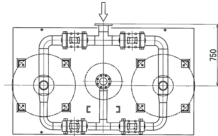
A-A詳細
